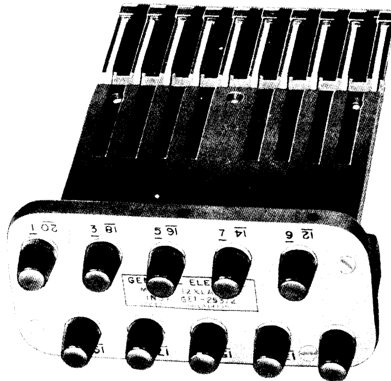
Fig. 2 XLA13A Test Plug
